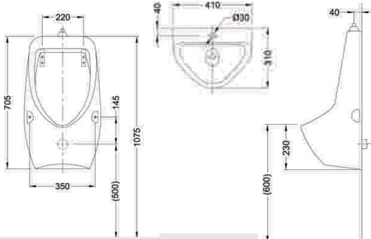
C2504W 310 X 400 X 705 mm
