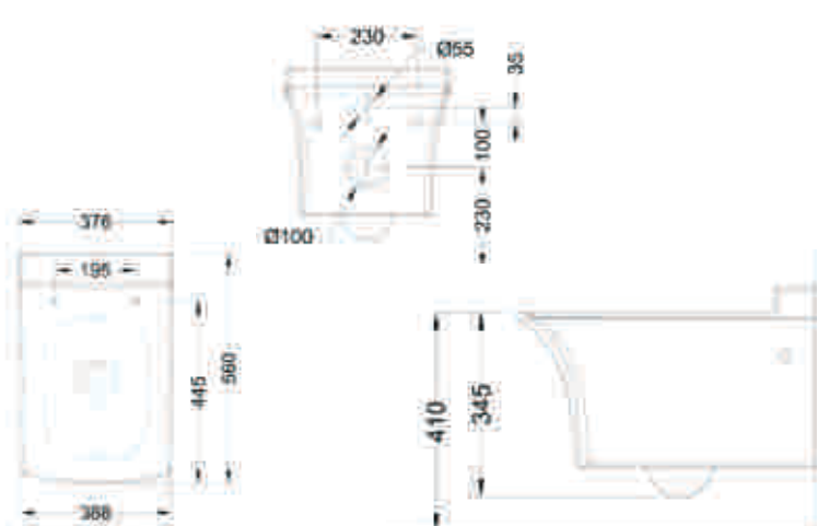
Philis Toilet C21104W 560 X 376 X 345
