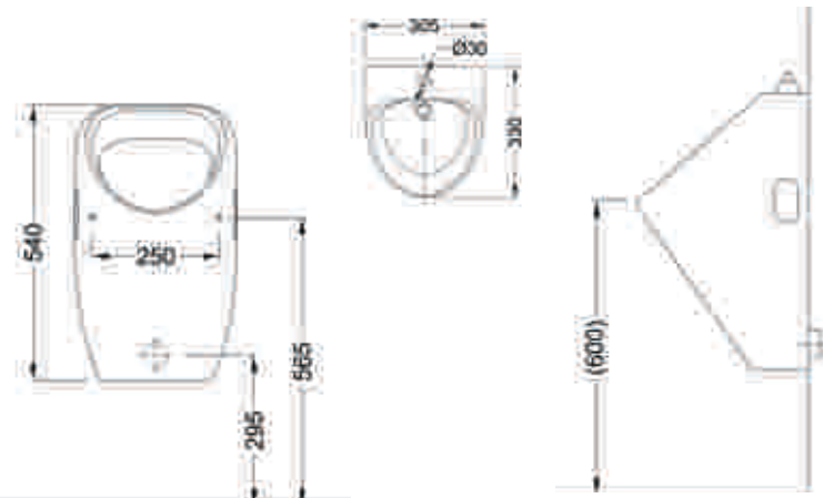
C2512W 330 X 305 X 540 mm
